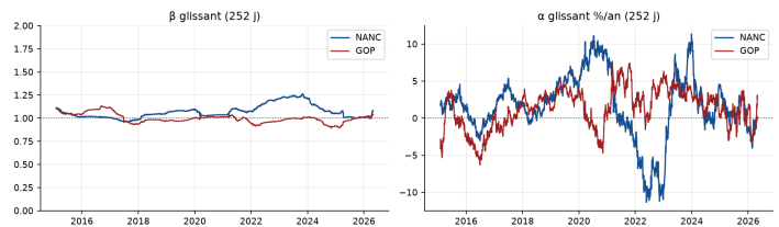
β et α glissants (OLS 252 j, validé = polyfit) : β colle à ~1 ; l'α traverse zéro sans cesse.
